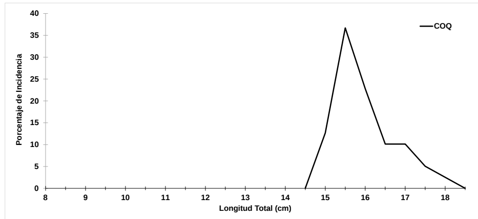
Figura 1. Estructura de talla del viaje muestreado en la región de Coquimbo, zona centro norte.
